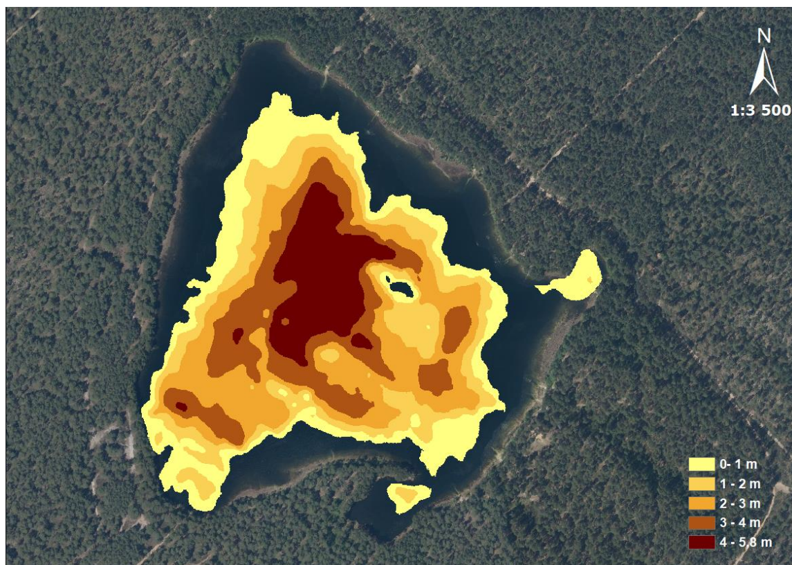
12.attēls. Ummja ezera nogulumu slāņa biezuma karte.
