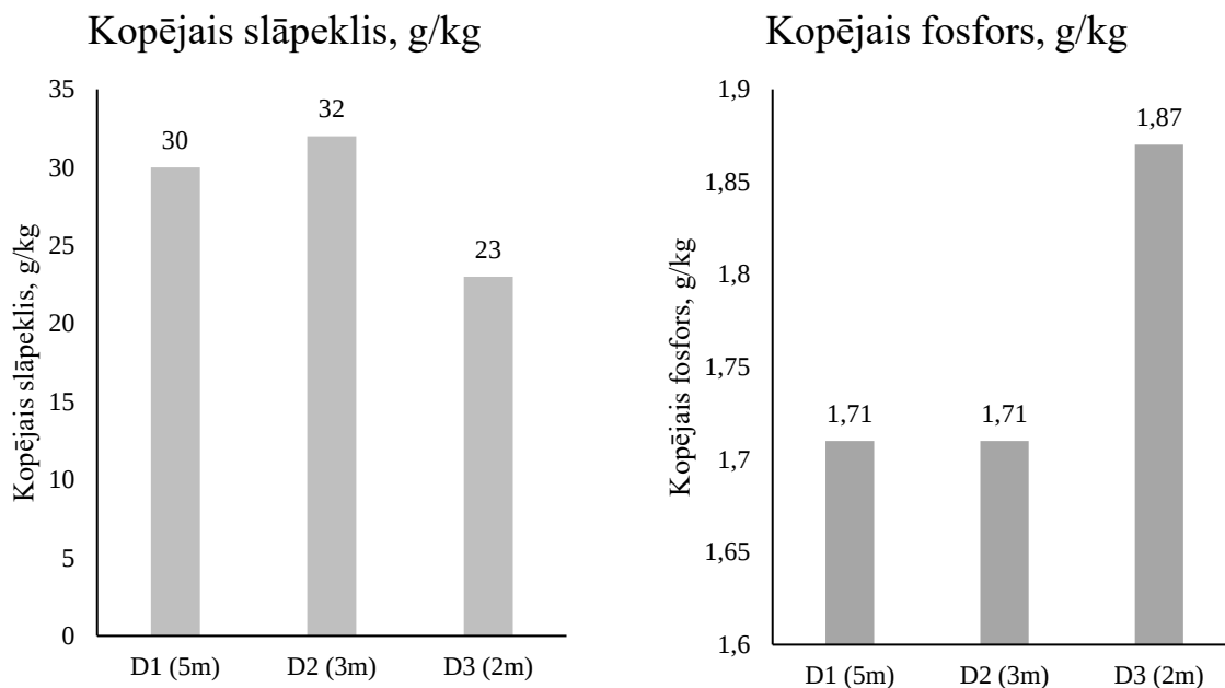
14.attēls. Kopējā slāpekļa un kopējā fosfora daudzums Ummja ezera dūņās 2021.gadā.
