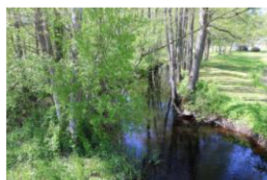
Podvāzes dabiskais tecējums lejpus AS "Latvijas valsts meži" ceļa starp Priekulānu un Klaucānu ezeriem (Foto J. Soms)
