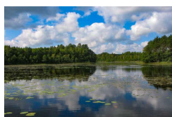
3150 Eitrofi ezeri ar iegrimušo ūdensaugu un peldaugu augāju
