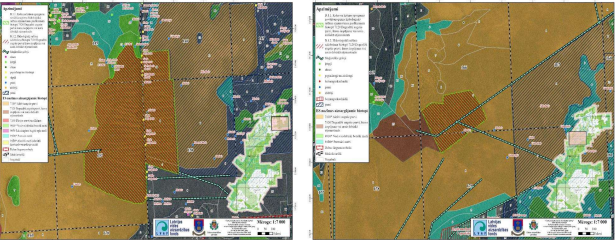
Hidroloģiskā režīma uzlabošanas poligoni biotopā 7120 Degradēti purvi, kuros iespējama vai noris dabiskā atjaunošanās
