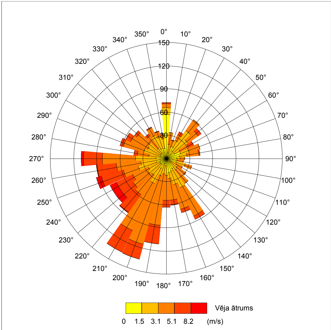
Vēja virzienu atkārtotāšanās 2007. gada ziemā
