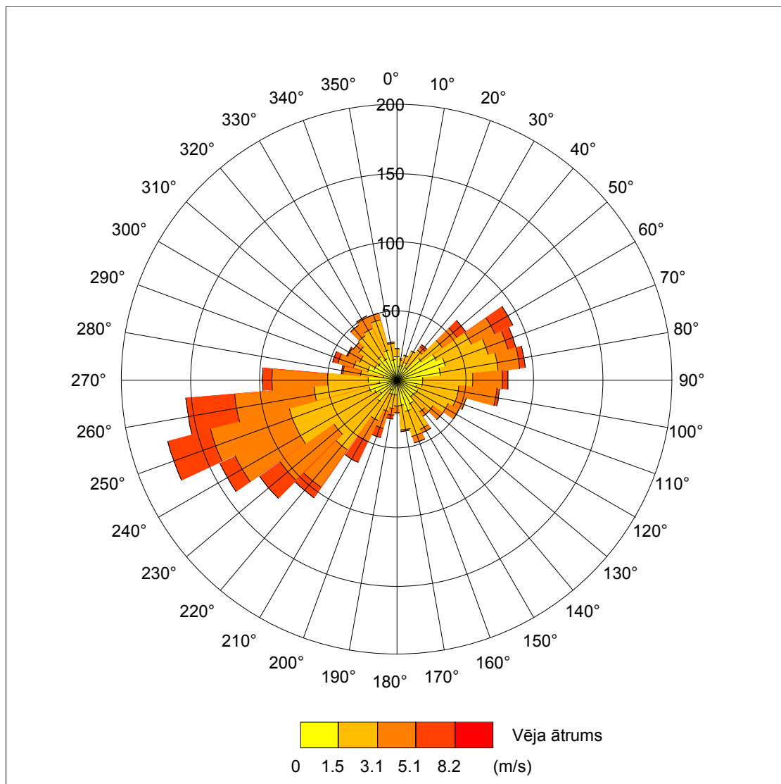
Vēja virzienu atkārtotāšanās 2007. gada vasarā
