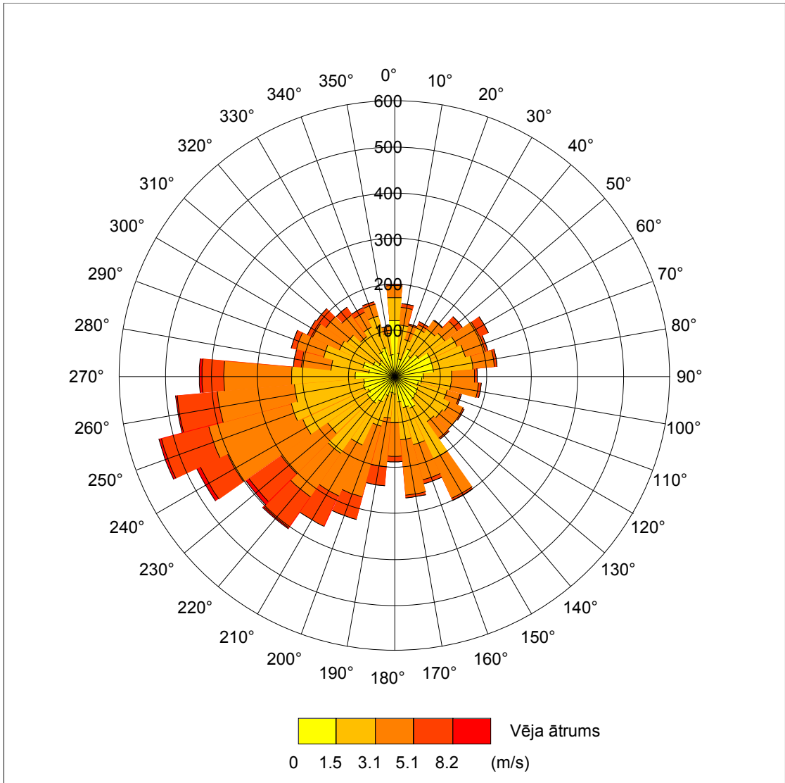
Vēja virzienu atkārtošānās 2007. gadā
